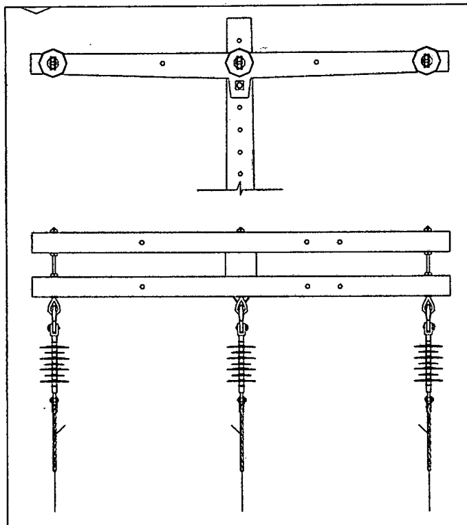
DETALHE FIM DE LINHA ESC.: ——— S/E
