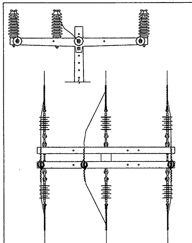
DETALHE ANCORAGEM DUPLA ESC.: ——— S/E
