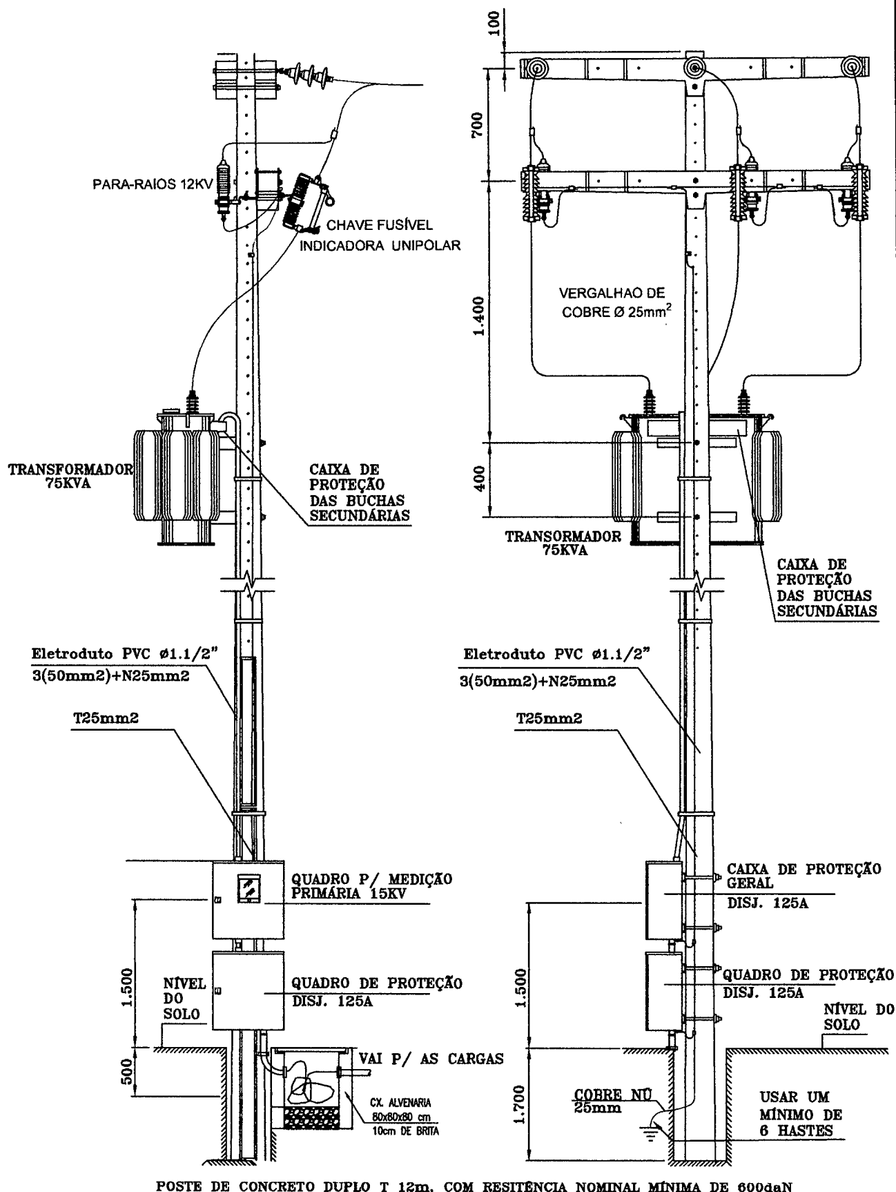
DETALHE DA SUBESTAÇÃO AÉREA (75KVA) VISTA FRONTAL E LATERAL ESC.: 1/50
